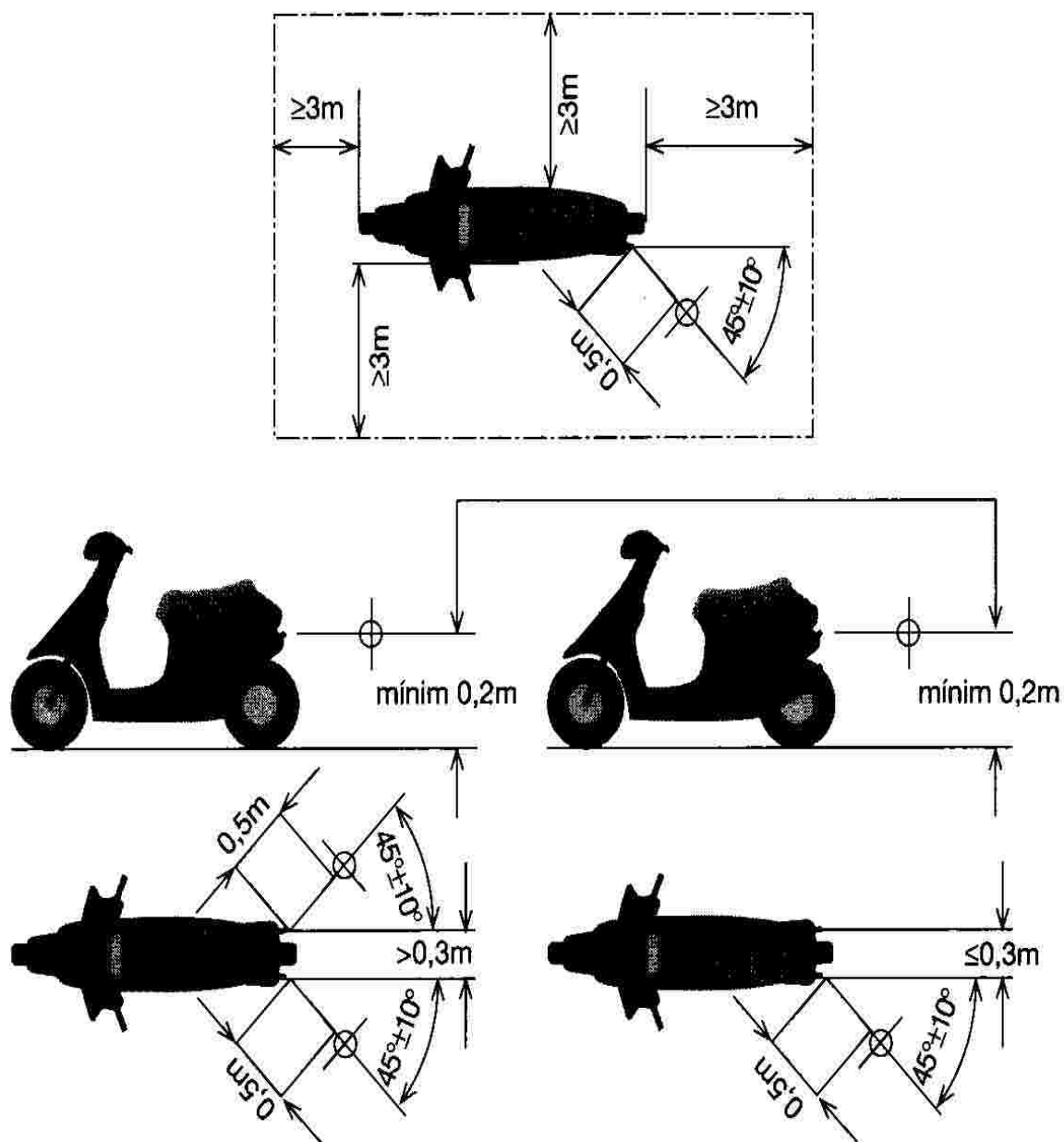
Figura 1. Posició de l'instrument de mesurament en ciclomotors, motocicletes i quadricicles
