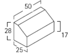
v25 central para bordillo t3 50 x 25 x 28 cm
