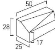
v25 lateral derecho para bordillo t3 50 x 25 x 28 cm
