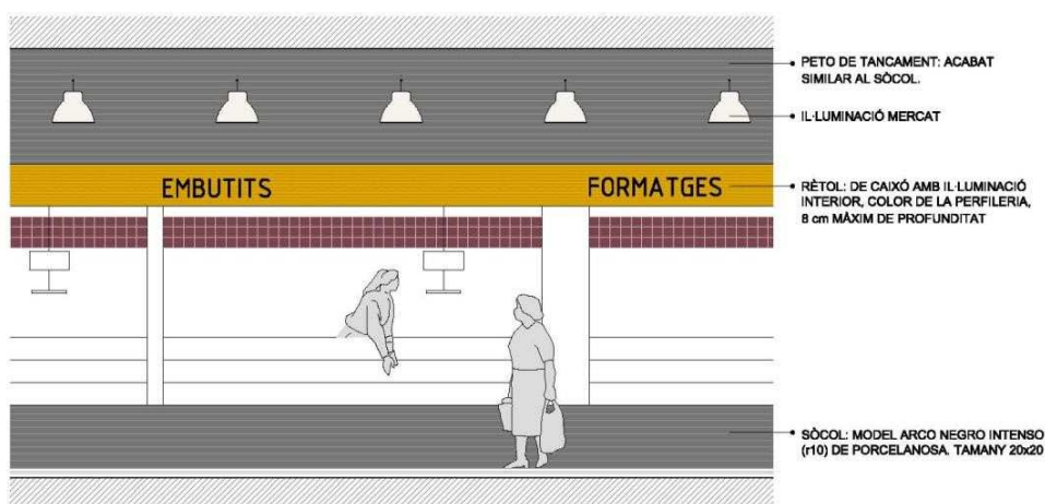
ALÇAT PARADES 1/50
