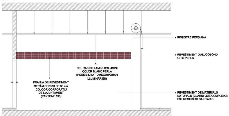
SECCIÓ PARADES 1/50
