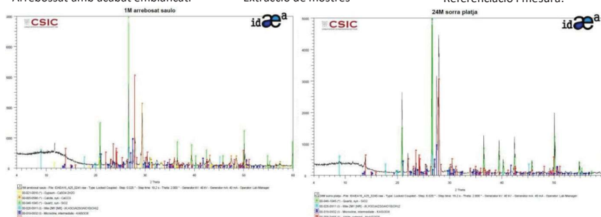
1.- Difractograma d'un arrebossat masnoví.
