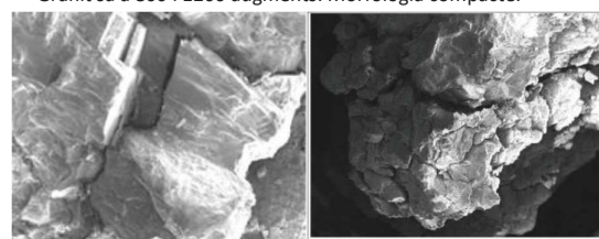
Granit degradat a 800 i 1200 augments: Morfologia esponjosa.
