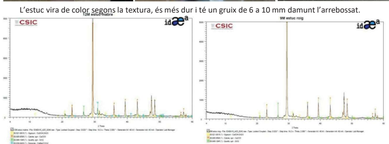
3.- Difractograma d'un estuc masnoví.
