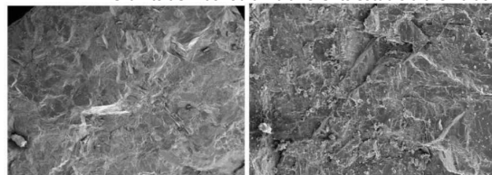
Granit sà a 800 i 1200 augments: Morfologia compacte.
