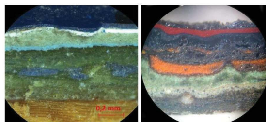
Micrografies de fusteria (esquerra) i de serralleria (dreta) a més augments (de 40 a 80) necessàries per apreciar les diferents capes i el seu color.
