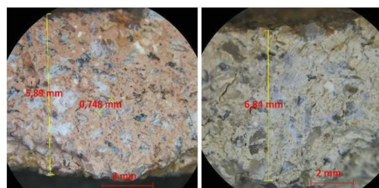
Micrografies d'estucs tenyits en massa a 10 augments.
